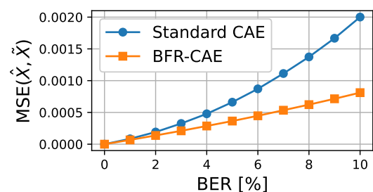
図2 bpp=2 における BER と MSE(\hat{X}, \tilde{X}) の関係
