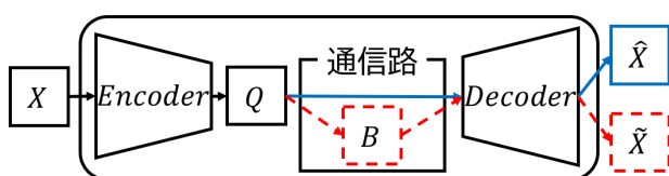
図1 BFR-CAE のモデル構造
